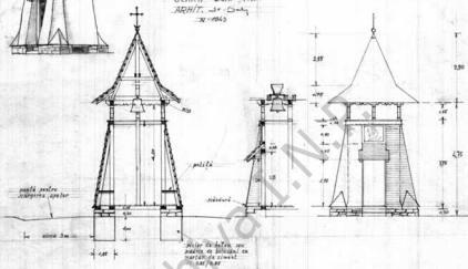
SECȚIE A-B
