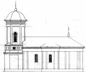
FĂȚADA LATERALĂ
