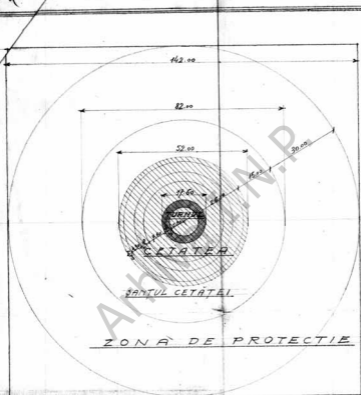
PLANUL SCHEMATIC AL CETATEI TURMU MAGURELE - SCARA 0 o 002 = 1 METRU
